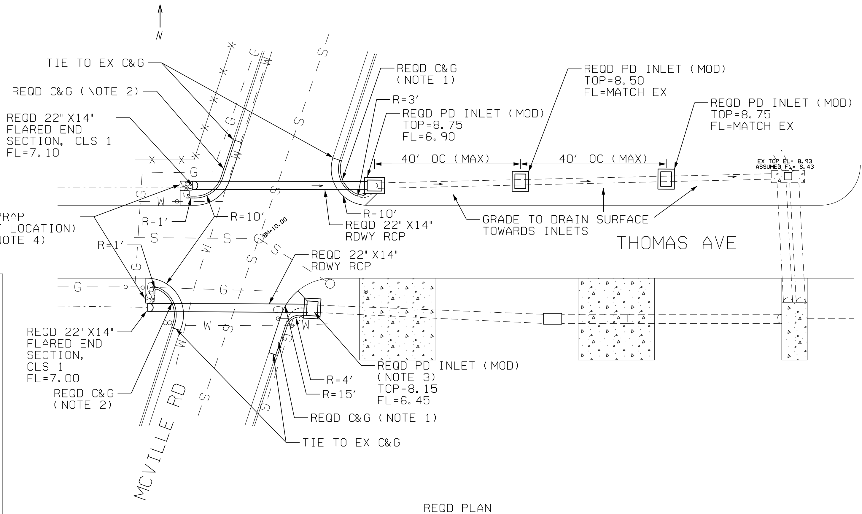
REQD PLAN
